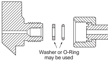
CGA 180 .625-18UNF-2A-RH-EXT
