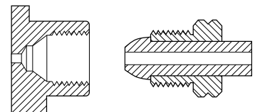
CGA 510 .885-14NGO-LH-INT (Bullet Nipple)
