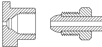
CGA 500 .885-14NGO-RH-INT (Bullet Nipple)
