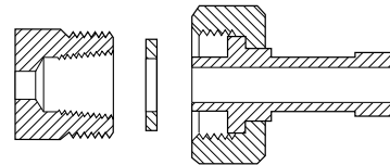
CGA 705 1.125-14UNS-2A-RH-EXT
