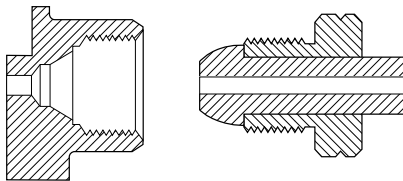
CGA 590 .965-14NGO-LH-INT
