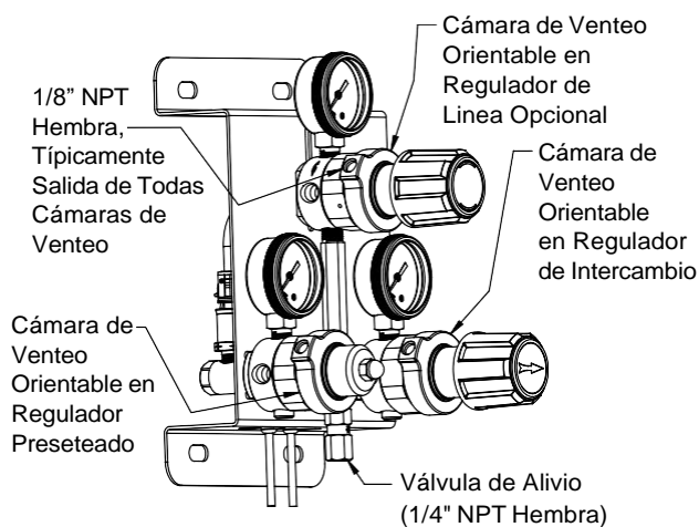
Figure 2 - Localización de la Válvula de Alivio
